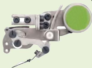
拨线器 Wiper
