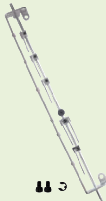
松线组件 Tension Disc Separator
