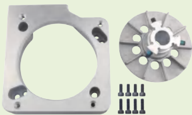
电机座子组件 Motor seat assembly
