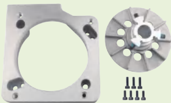
电机座子组件 Motor seat assembly
