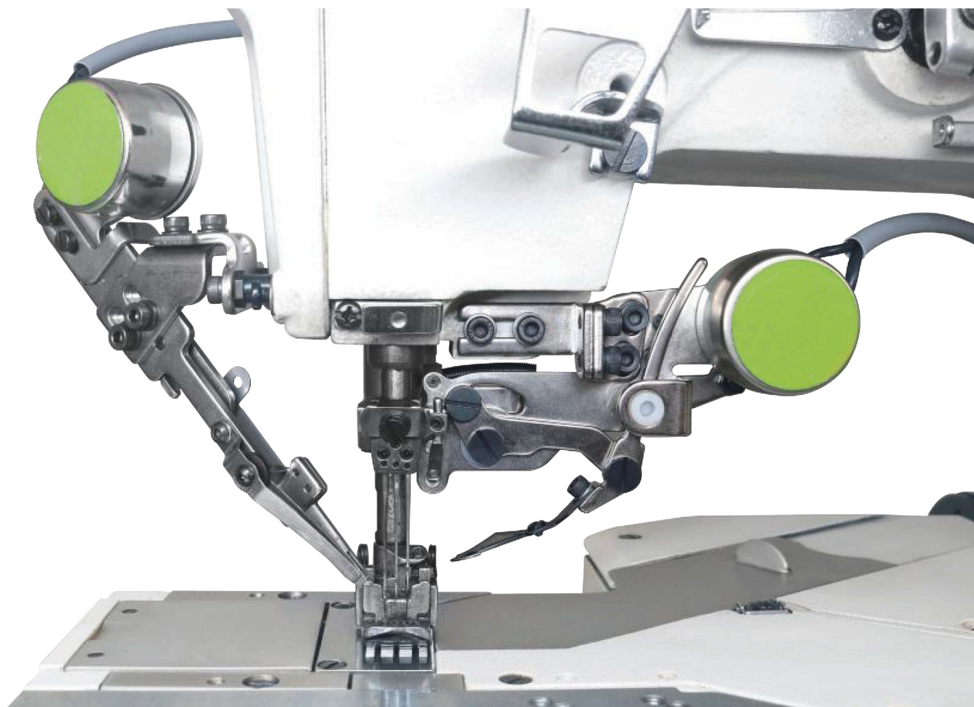
拨线器 Wiper
